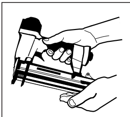
3. Pousser le magasin vers l'avant.
